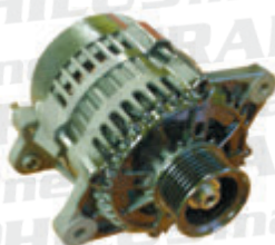
Alternator 12V, 70A za MerCruiser nove motore od 2002 do 2023, Delco (remenica Ø50mm)
