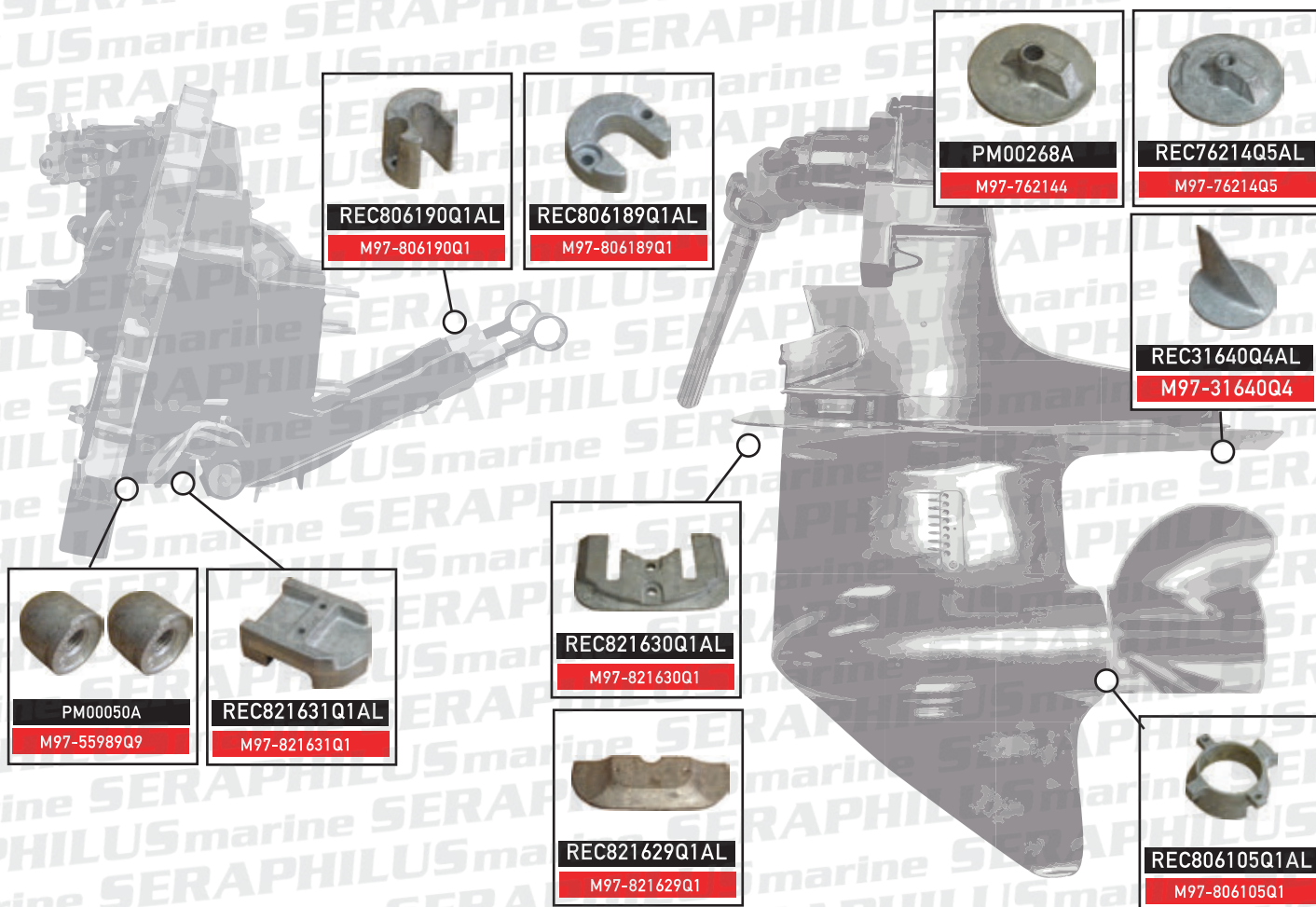
Anoda trim cilindra za MerCruiser Bravo
