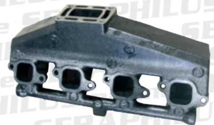
Ispušni kolektor za Volvo 7.4
